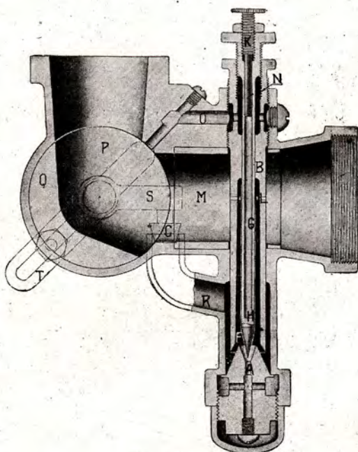
Corte longitudinal
